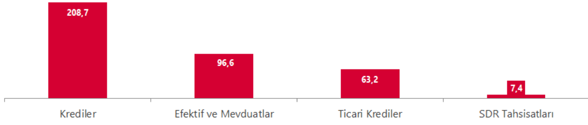
Grafik 4: Dięer Yatırım Yüklümlüklerinin Kompozisyonu (Stok, Milyar ABD Doları)
